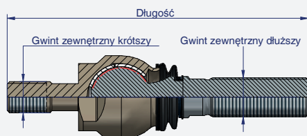
Przegub wzdłużny TYP 5
