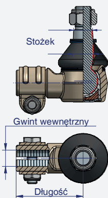
Przegub poprzeczny TYP 1
