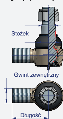
Przegub poprzeczny TYP 2
