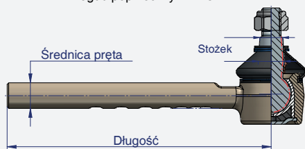
Przegub poprzeczny TYP 3
